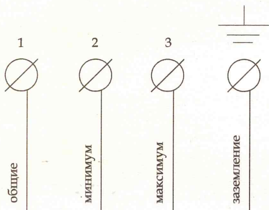
Рисунок 3 - Схема внешних электрических соединений
